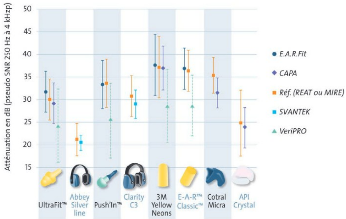
Document 4: Comparaison des atténuations mesurées selon les fabricants pour plusieurs dispositifs de protection auditives
